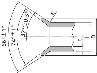
厚壁 Tube 管
