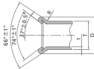
薄壁 Tube 管
