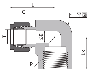
卡套阴螺纹弯头
