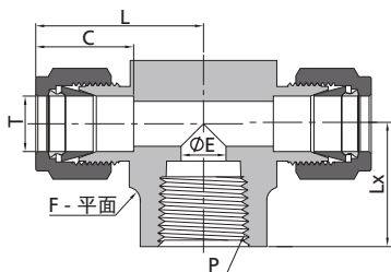
支管阴螺纹卡套三通
