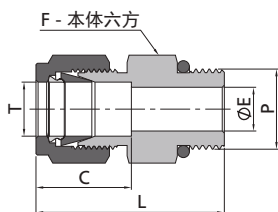
英制 Tube 管转 SAE/MS 直螺纹
