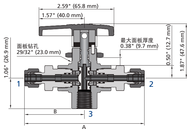
3 通阀
