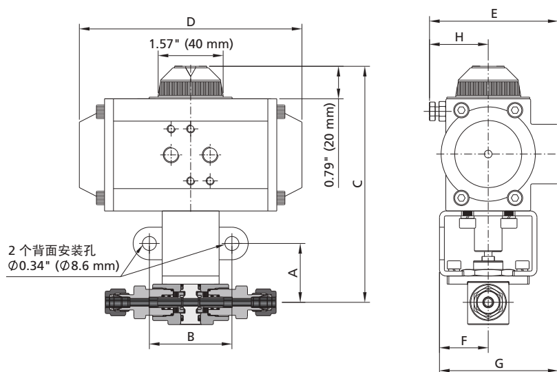
2 通阀
