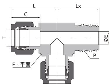
主管阳螺纹卡套三通
