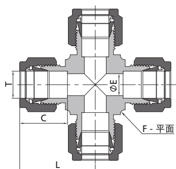
卡套四通
