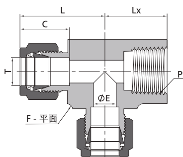
主管阴螺纹卡套三通
