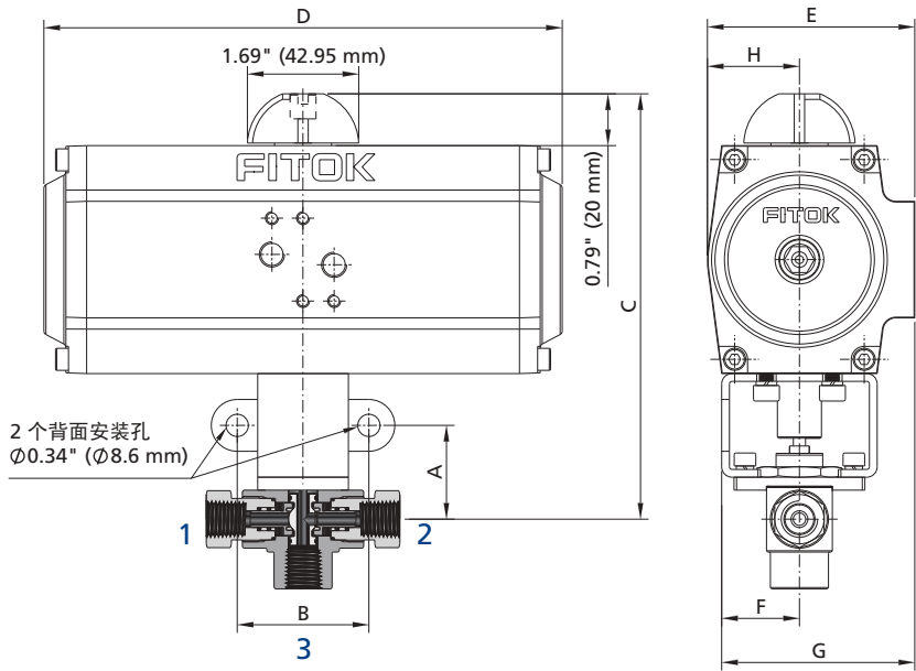
3 通阀
