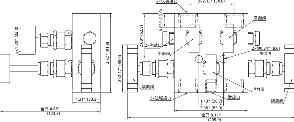
5R□□-FNS8-VB-E
