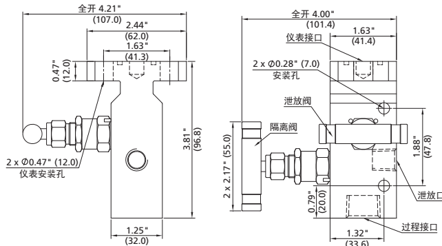
2D□□-FNS8-V
