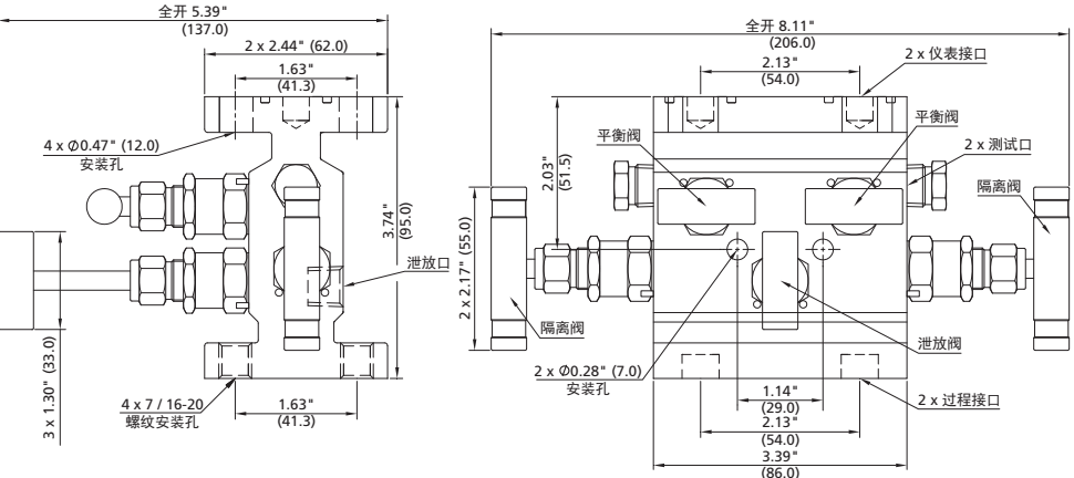
5D□□-F-VB-E
