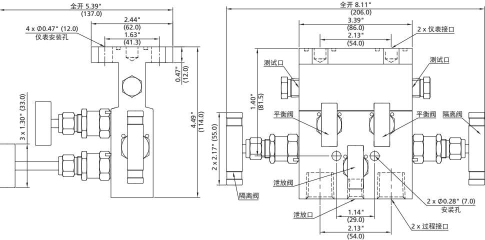
5D□□-FNS8-VB-E
