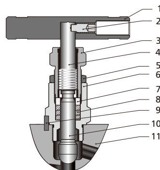
球头设计表阀 (GV、GVH)
