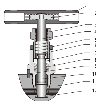
旋塞头设计表阀 (GR)
