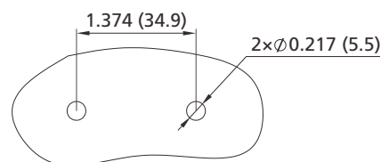
底部安装固定开孔
