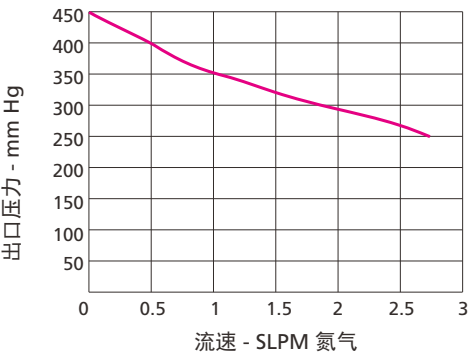
适用出口调压范围代码 V30 的阀门
