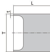
管外径 ≥ 1/2 in. 示意图
